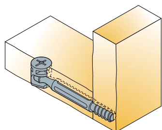
Cam2000 Ø12
